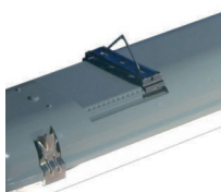
Löstagbara upphängningsbyglar
